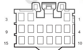
I_RRDB RR Door W.H. Connector Connecting Body W.H.
