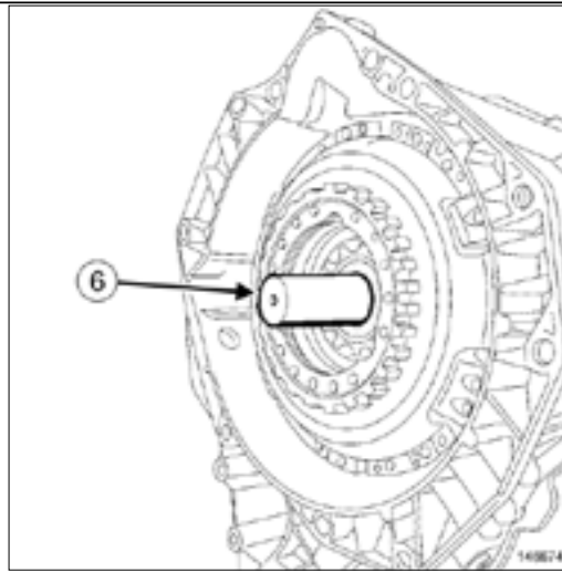
کاسه نمد شفت ورودی با قطر کوچک را با استفاده از ابزار باز کردن - نصب مجدد کاسه نمدهای شفت ورودی (DC4) (25412091) (۶) نصب کنید.
