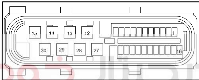
F11 Electronic Handbrake Module
