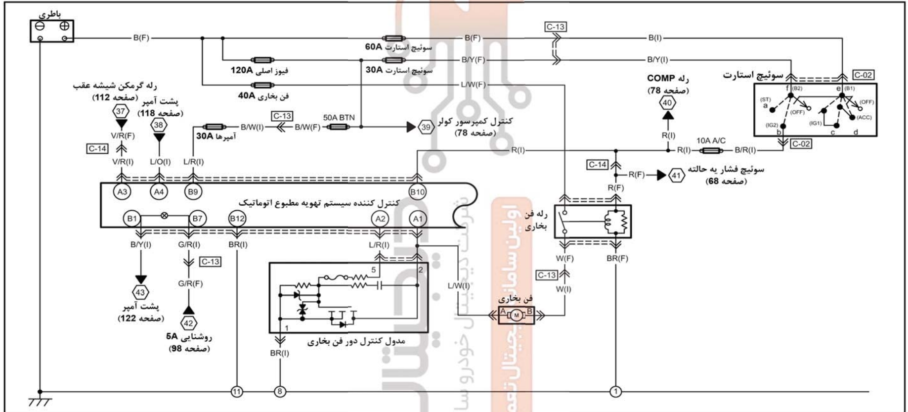
A سیستم تهویه مطبوع اتوماتیک
