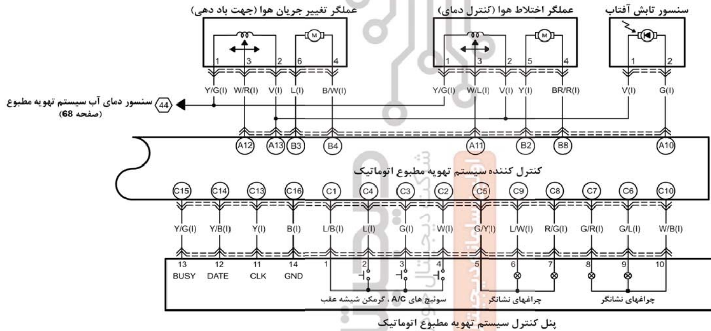
A سیستم تهویه مطبوع اتوماتیک
