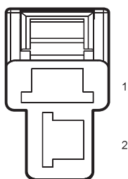
E29 Clutch Pedal Switch
