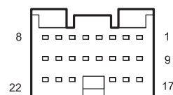
D14 Right Rearview
