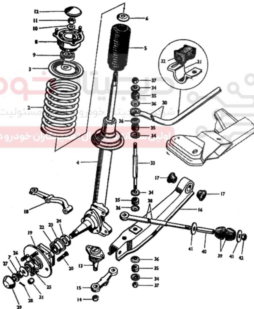
شکل ۱۱: میل موج‌گیر
