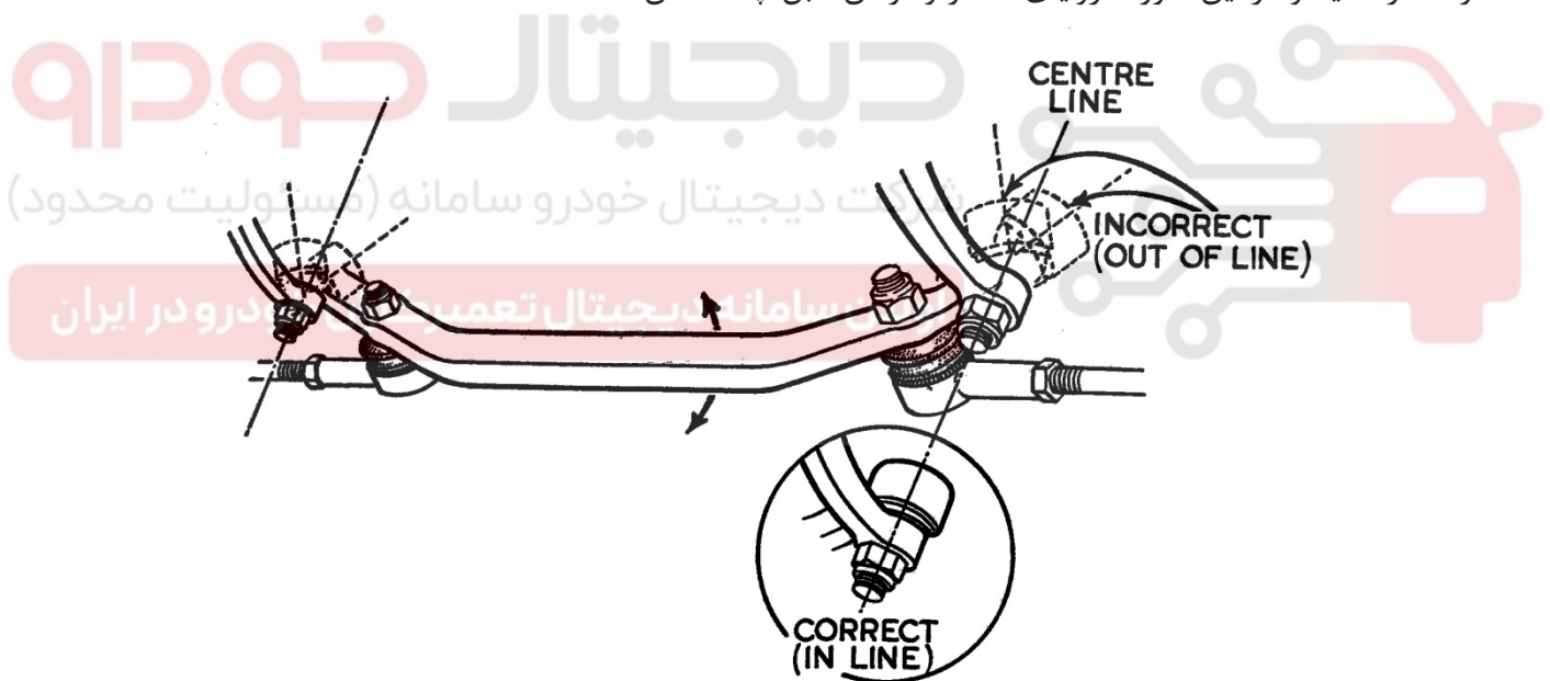
شکل ۶: تنظیم سیبک
