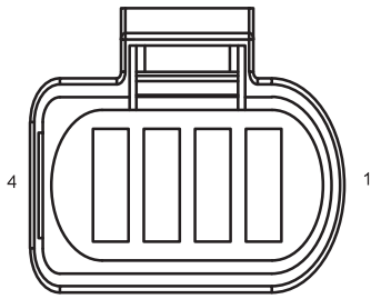
E12 Front Wiper Motor
