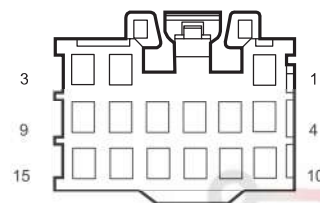
I_RRDB RR Door W.H. Connector Connecting Body W.H.
