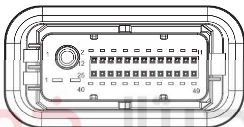
Body W.H. Connector Connecting FL Door W.H.
