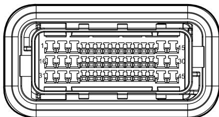
I_BFRD Body W.H. Connector Connecting FR Door W.H.
