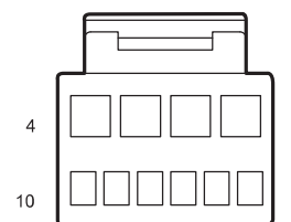
D05 FL Door Lock
