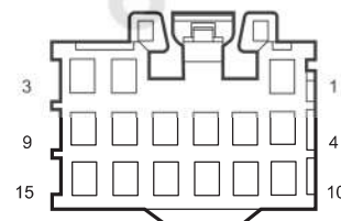
I_RLDB RL Door W.H. Connector Connecting Body W.H.
