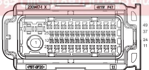
FL Door W.H. Connector Connecting Body W.H.
